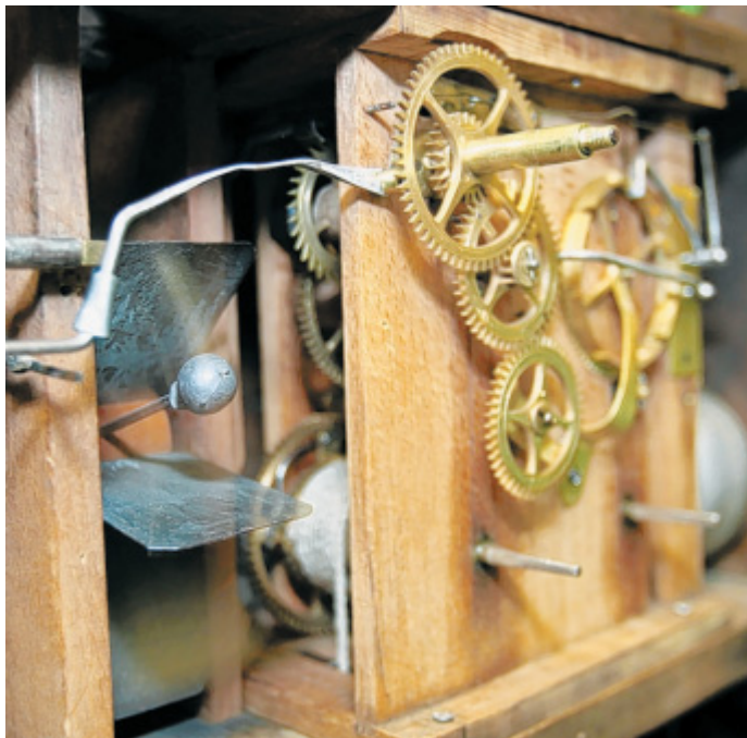
Zahn in Zahn: Herzstück der Flötenuhr ist ein konventionelles Pendel-Uhrwerk mit Zahnrädern aus Messing.
